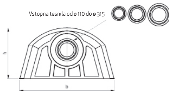
Tehnična skica vstopnega priključka tunela
